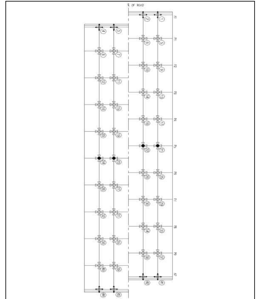
【그림 5.2.14】 받침배치현황(부산)
