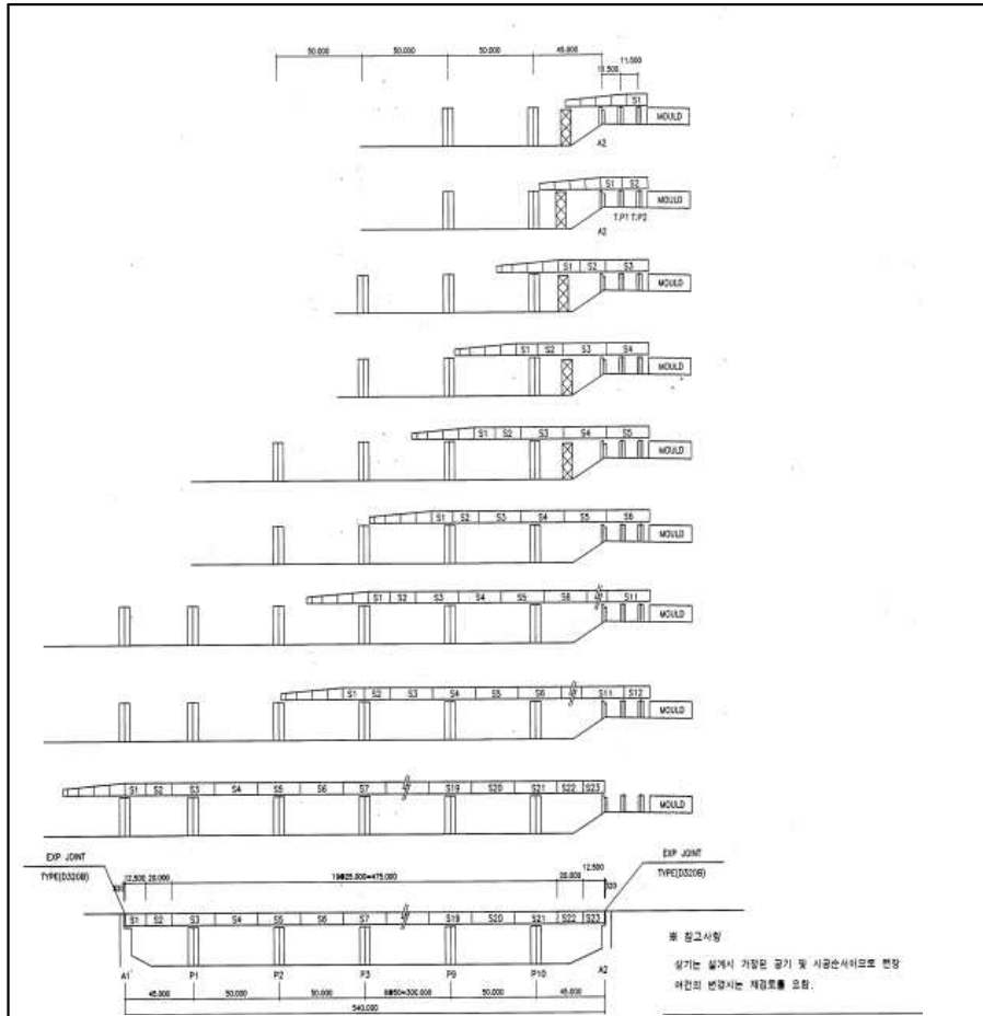
<시공 순서도>
