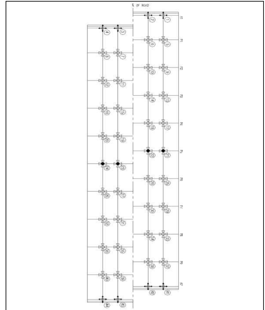
【그림 5.2.1】 받침배치현황(대구)
