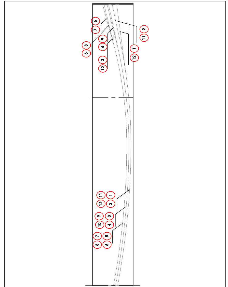
【그림 5.2.7】 강선배치 개요도(대구)
