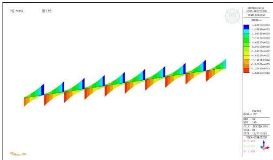
【그림 5.2.9】 활하중에 의한 부재력(대구)
