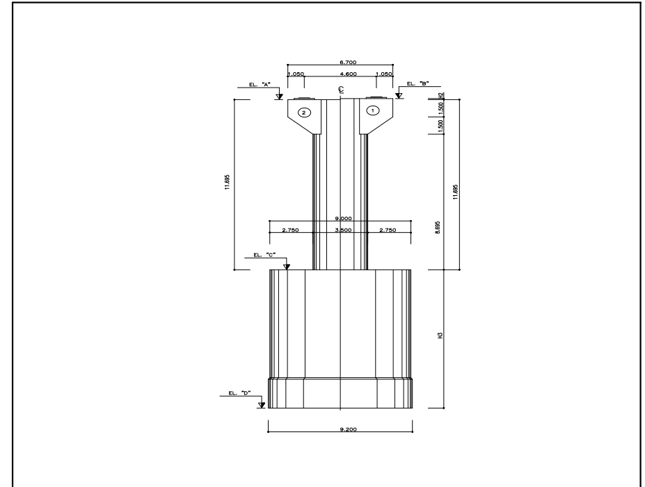
【그림 5.4.12】 해석단면(P5)(부산)
