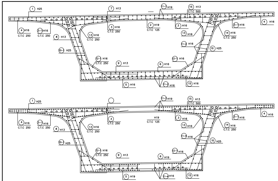
【그림 5.2.13】 배근도, TYPE 1, TYPE 2(대구)
