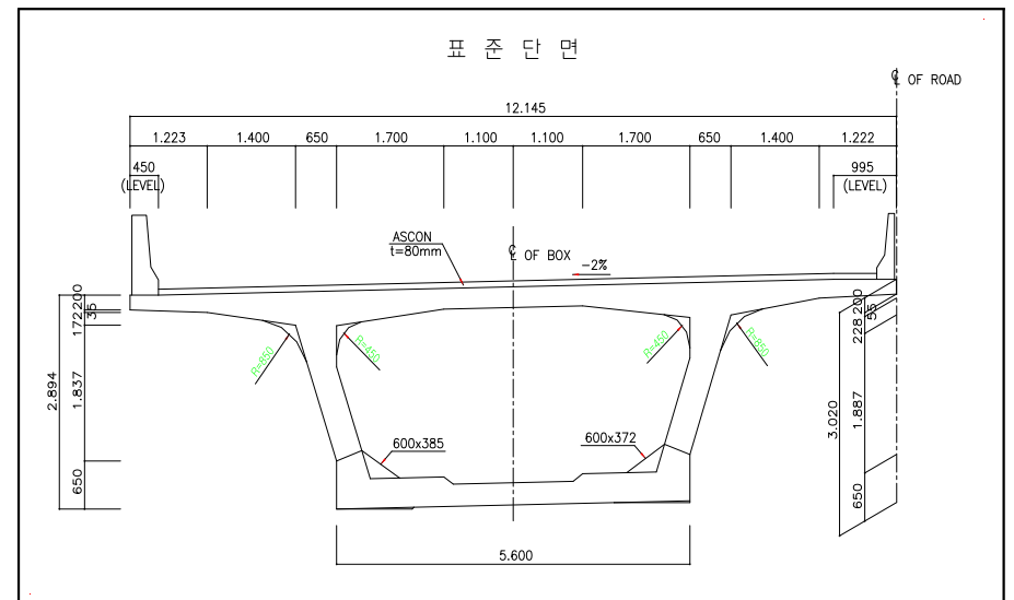
【그림 5.2.5】 구조해석 단면제원(대구)
