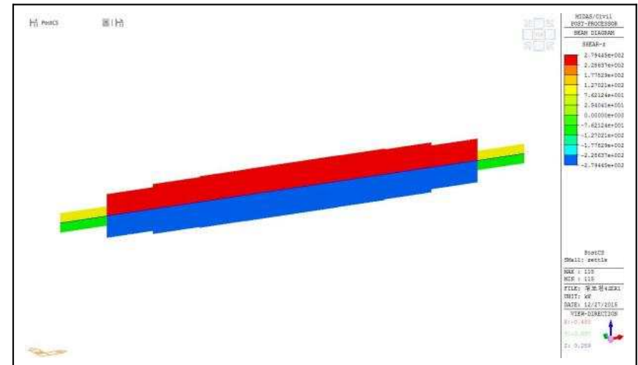
【그림 5.2.10】 지점침하에 의한 부재력(대구)
