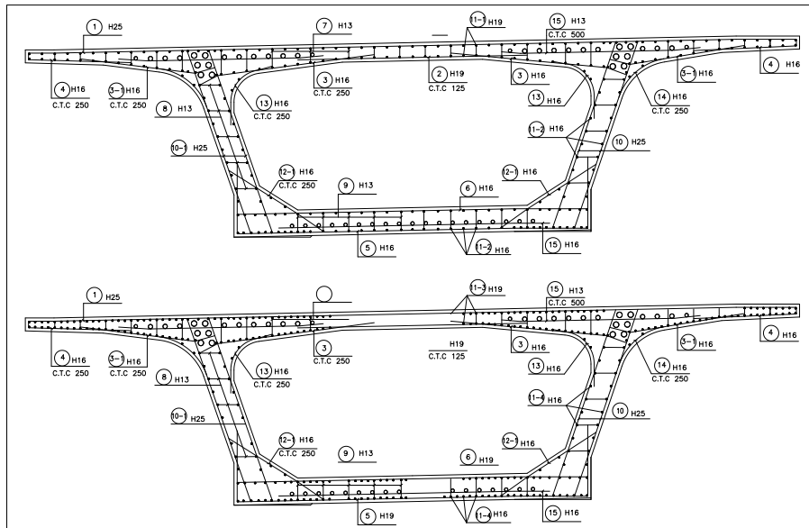
【그림 5.2.26】 배근도, TYPE 1, TYPE 2(부산)
