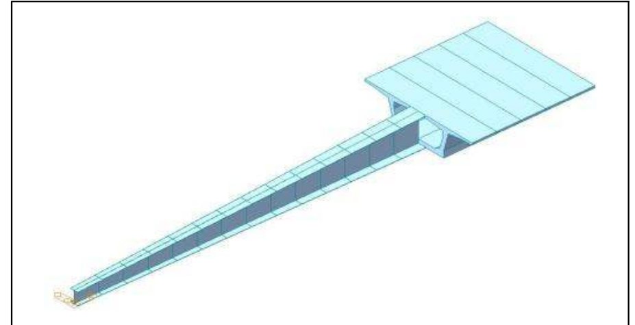
【그림 5.2.4】 압출노즈 모델링도(CS1)(대구)
