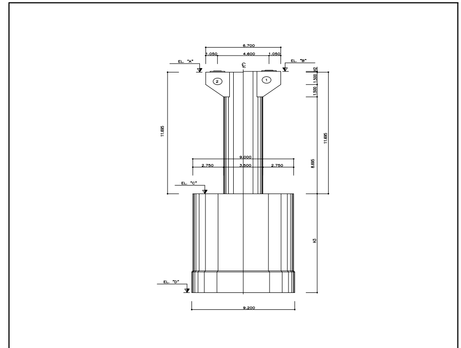
【그림 5.4.1】 해석단면(P5)(대구)
