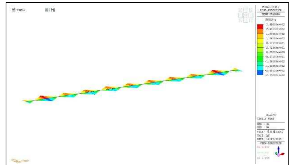
【그림 5.2.12】 풍하중에 의한 부재력(대구)
