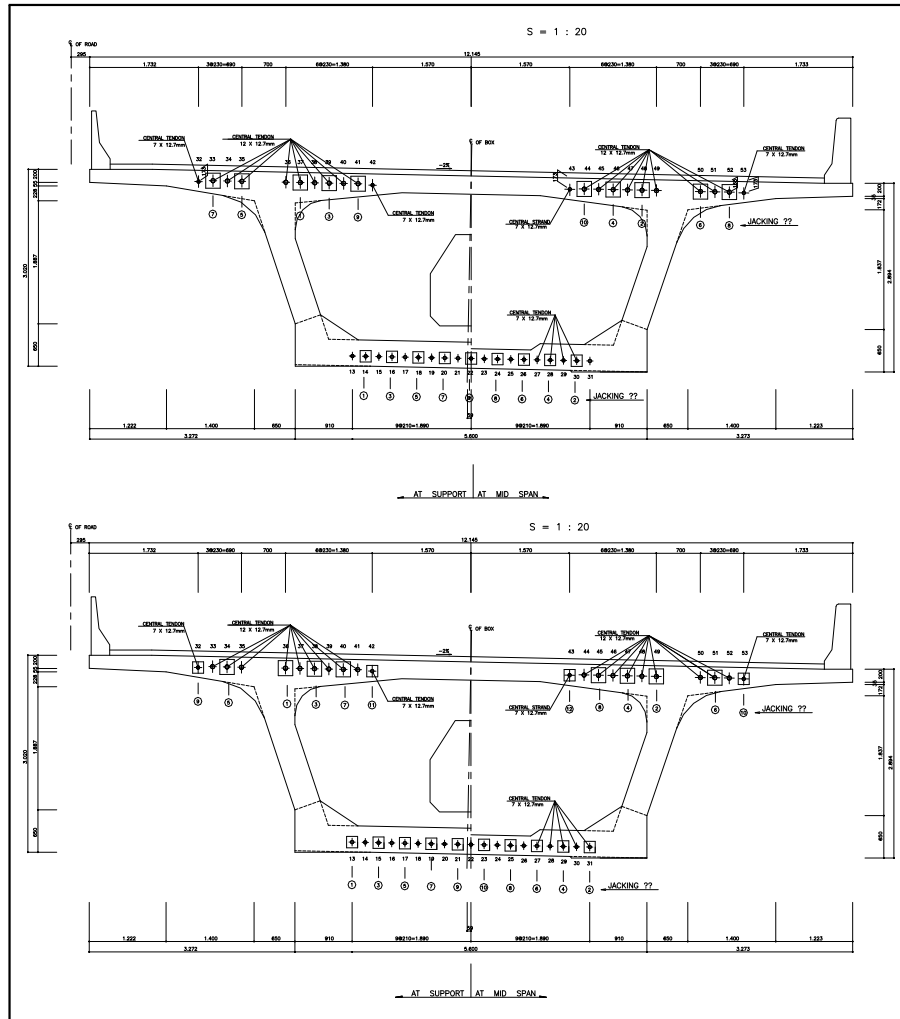
【그림 5.2.19】 구조해석 단면제원강선 배치도(부산)
