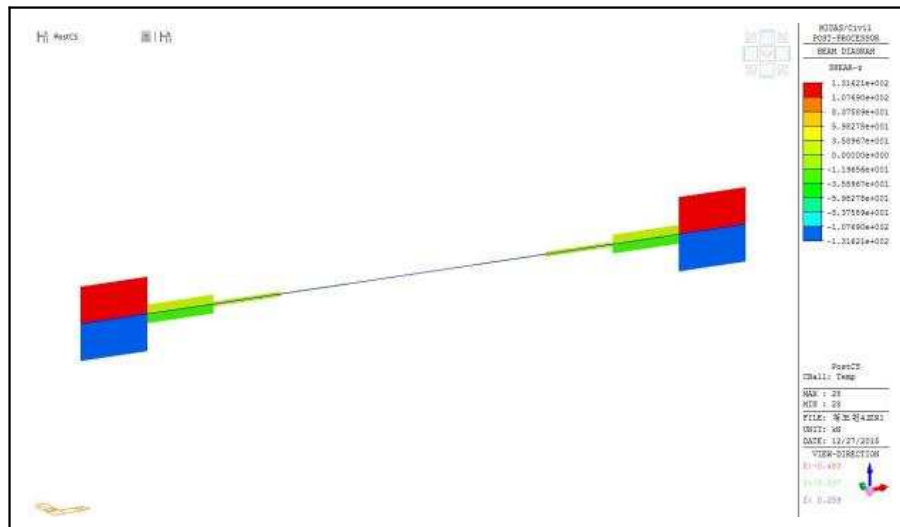
【그림 5.2.11】 온도 하중에 의한 부재력(대구)
