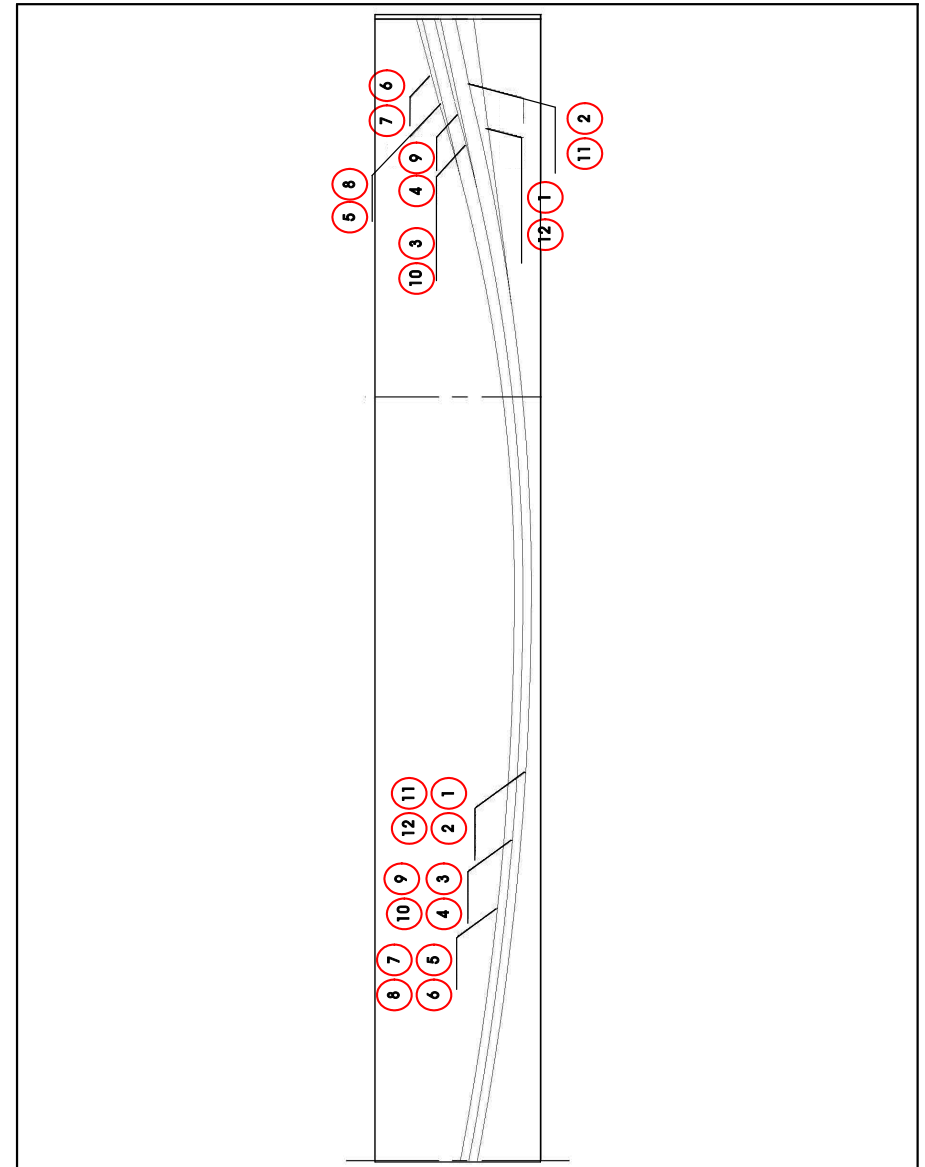
【그림 5.2.20】 강선배치 개요도(부산)
